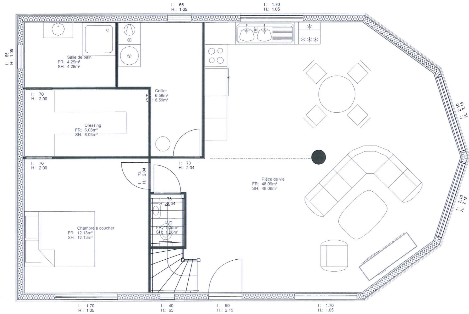
Oriane 5 pans Rez-de-chaussée Echelle : 1/50
