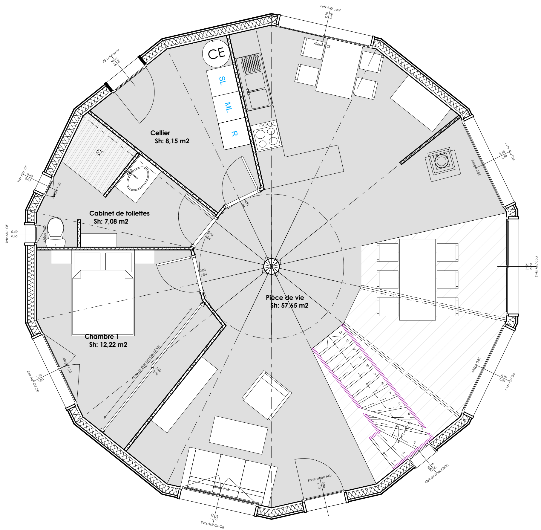
Rez de Chaussée
